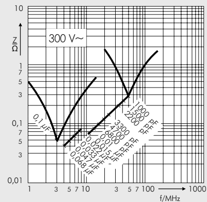
Scheinwiderstand in Abhängigkeit von der Frequenz (Richtwerte)
